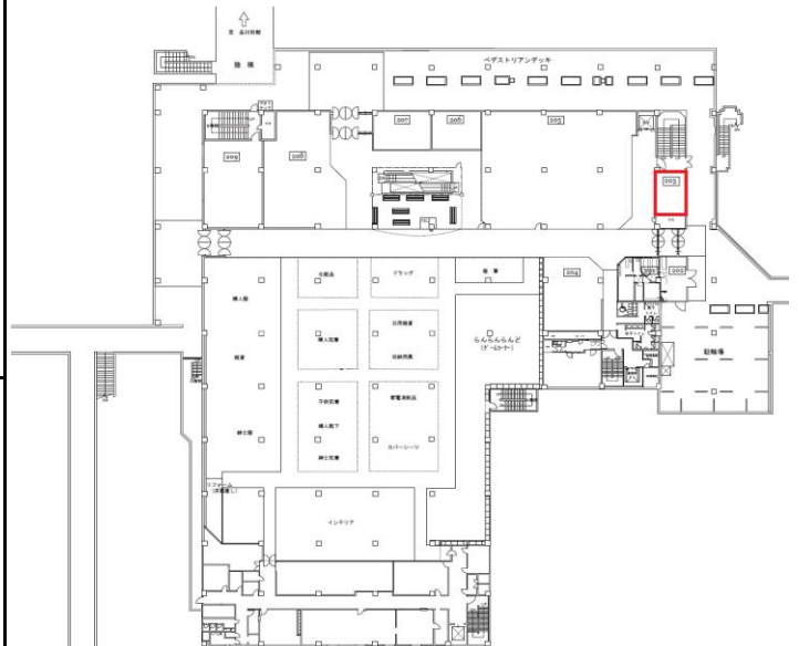
【2階平面図】
